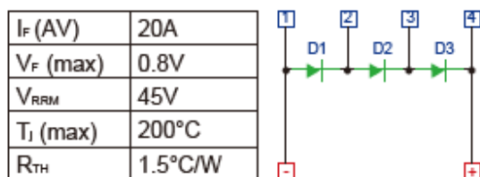
Specyfikacja i konfiguracja diody
