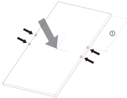
Rys. 7 Rodzaj śrubowania
