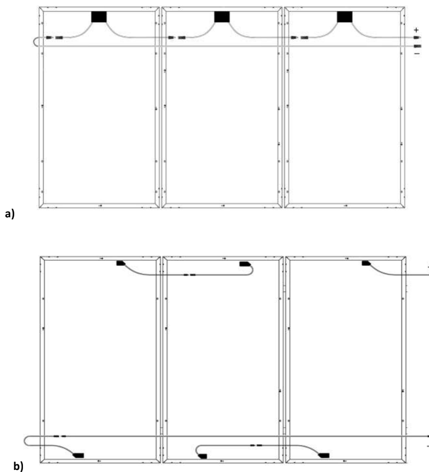
Rys. 2. Zalecane sposoby prowadzenia przewodów w instalacjach PV: a) moduły standardowe, b) moduły typu 'half cut'
