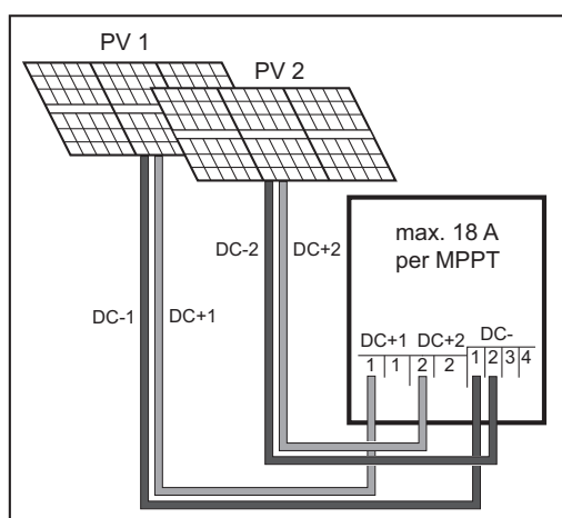
Podłączenie dwóch łańcuchów modułów solarnych do falownika typu Multi MPP Tracker
