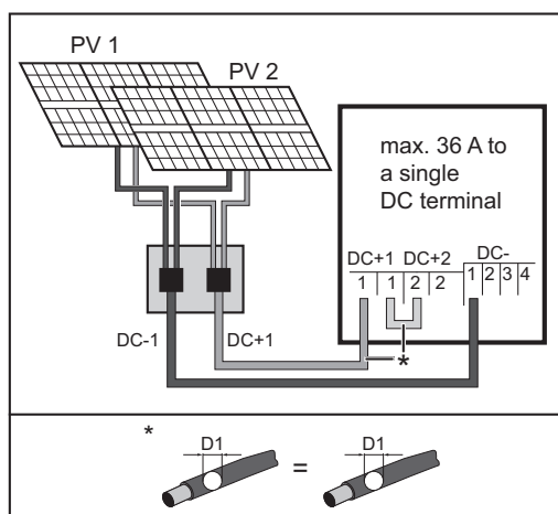
Podłączenie większej liczby połączonych ze sobą pół modułów solarnych za pomocą jednego przewodu do falownika typu Multi MPP Tracker
